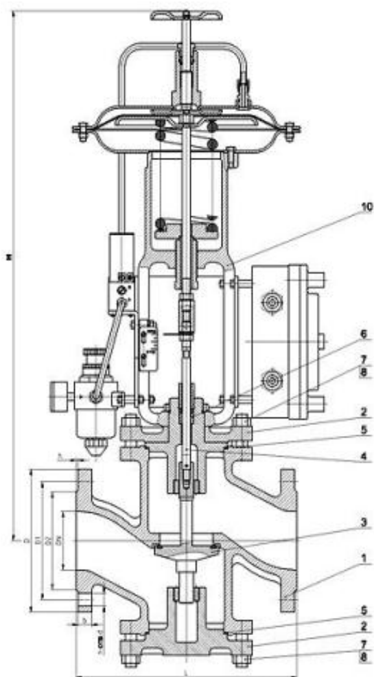
Клапан отсечной сальниковый
