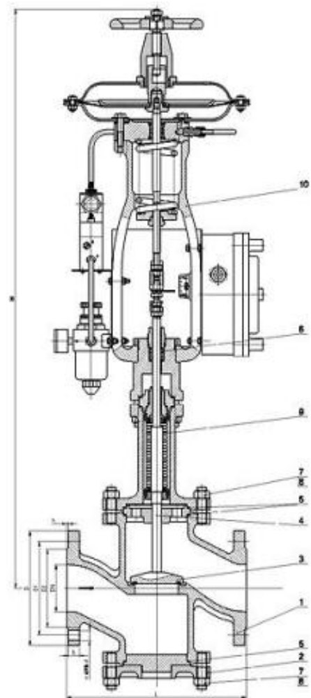
Клапан отсечной сильфонный
